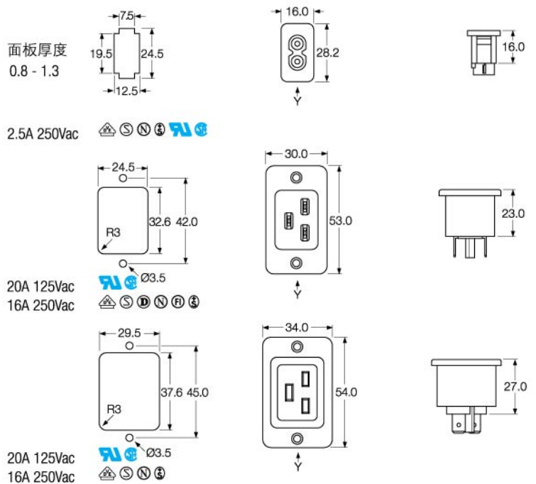
尺寸图 (mm)
