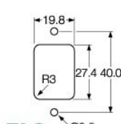
尺寸图 (mm)
